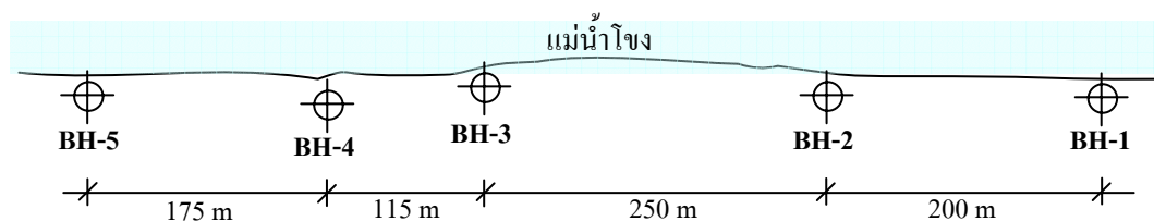
รูปที่ 9 แผนผังตำแหน่งหลุมเจาะ
