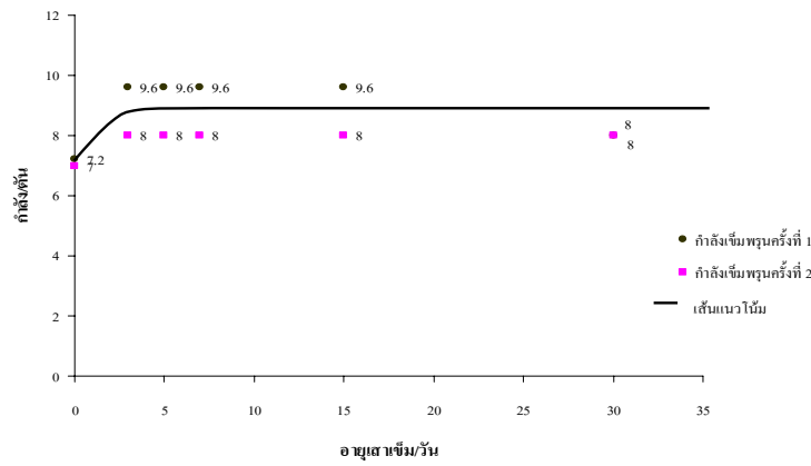
รูปที่ 12 กราฟค่าเส้นแนวนอนระหว่างเวลา กับ น้ำหนักบรรทุก ของเข้มนวพูน
