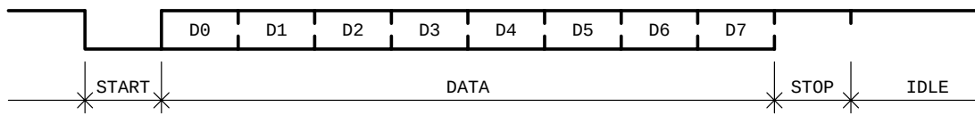
รูปที่ 9 ช่วงเวลาการสื่อสารอนุกรมแบบ UART
