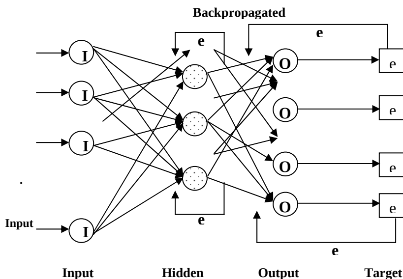
รูปที่ 2 โครงข่าย MLFF สำหรับโครงสร้าง Backpropagation
