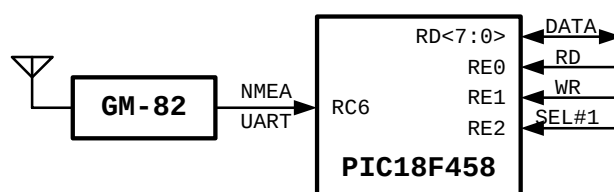
รูปที่ 8 ผังวงจรหน่วยคำนวณตำแหน่ง
