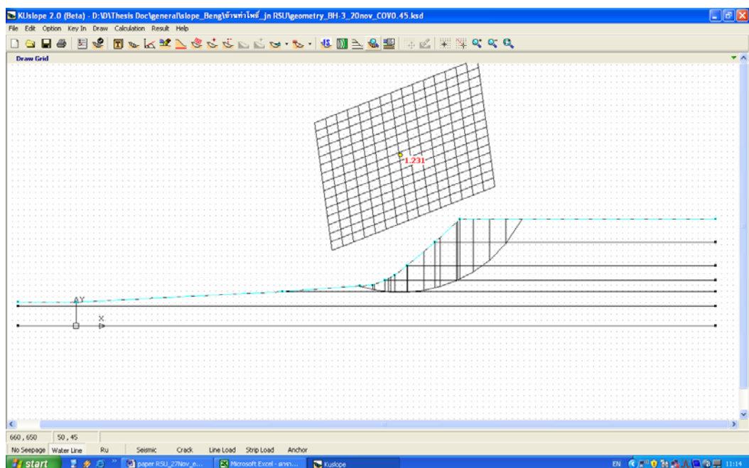
รูปที่ 8 รูปแบบการพิบัติของลาดดิน
