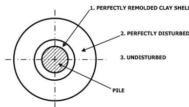
รูปที่ 1 แสดงขอบเขตการรบกวนของดินรอบๆเสาเข็ม
