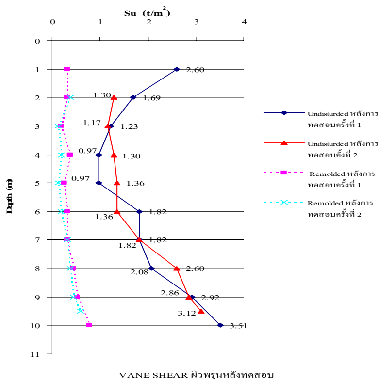
รูปที่ 14 กราฟผลการทดสอบกำลังแรงเฉือนดินเสาชี้มพูน หลังการทดสอบ ครั้งที่ 1 และ 2
