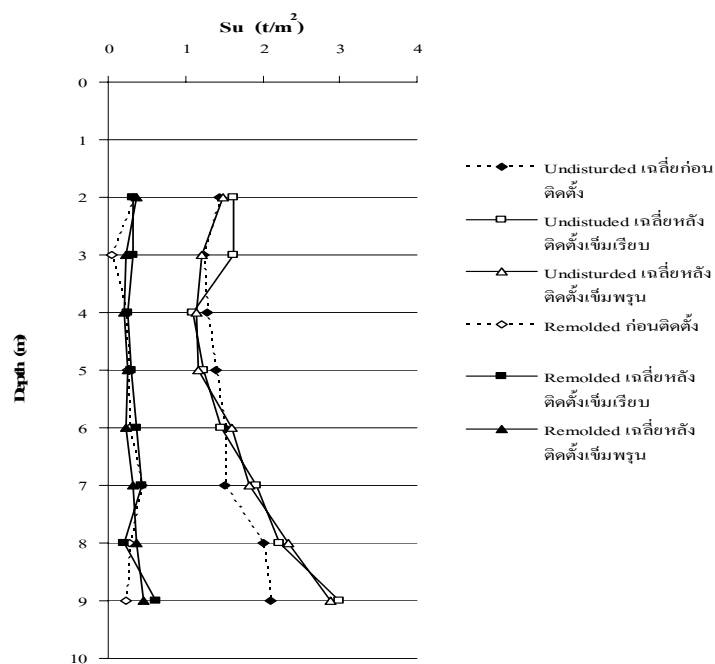
รูปที่ 15 กราฟผลการทดสอบกำลังแรงเฉือนดินเสาเข็มเรียบ หลังการทดสอบ ครั้งที่ 1 และ 2
