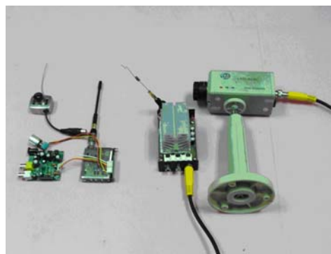
รูปที่ 14 ชุดส่งสัญญาณวีดีโอสำหรับหุ่นยนต์บิน
