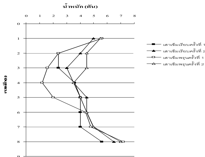
รูปที่ 8 กราฟแสดงค่าแรงกดในการติดตั้งเสาเข็ม
