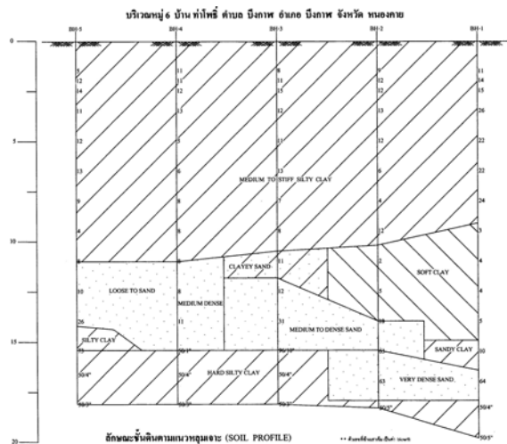
รูปที่ 5 ลักษณะชั้นดิน (Soil profile) บ้านท่าโพธิ์ อ.บึงกาฬ จ.หนองคาย
