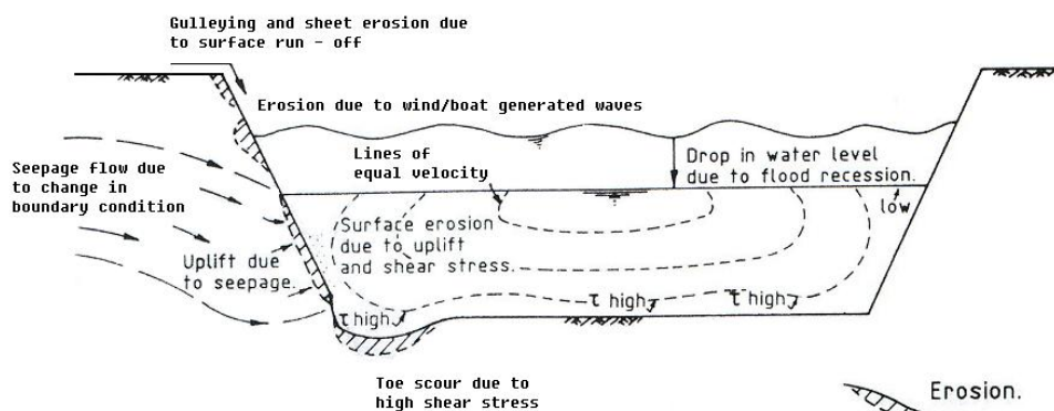
รูปที่ 1 กระบวนการทางกลศาสตร์ที่ทำให้เกิดการกัดเซาะ (IWEM, 1989)
