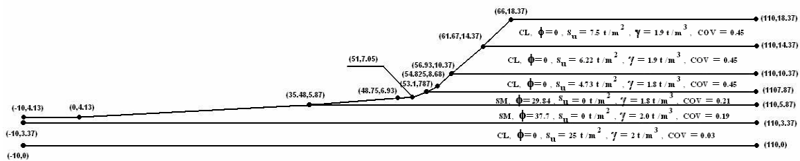
รูปที่ 6 ภาพตัดลาดดิน บ้านท่าโพธิ์ ม.6 อำเภอบึงกาฬ จังหวัดหนองคาย
