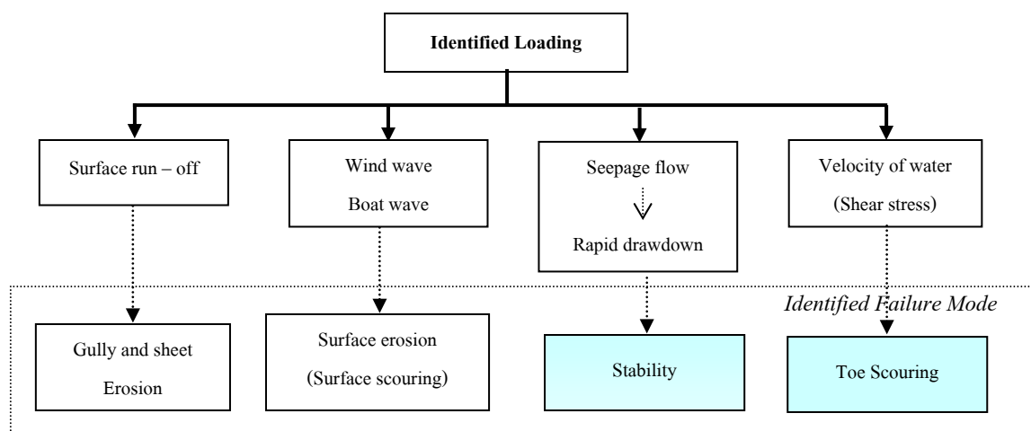
รูปที่ 2 แผนภูมิของแรงกระทำและรูปแบบการพิบัติ
