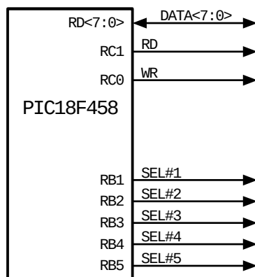
รูปที่ 6 ผังวงจรหน่วยควบคุมกลาง
