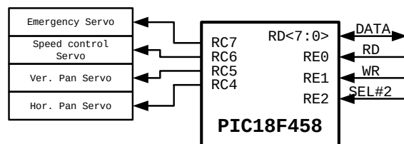
รูปที่ 12 ผังวงจรหน่วยขับเคลื่อน
