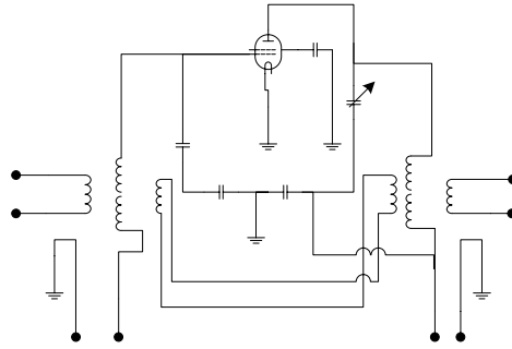
รูปที่ 3 วงจรชุดเซออุณหภูมิต
