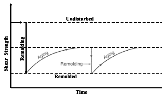
รูปที่ 2 กราฟแสดงการคืนกำลังของดินที่เกิดการคืนกำลังเพียงบางส่วน
